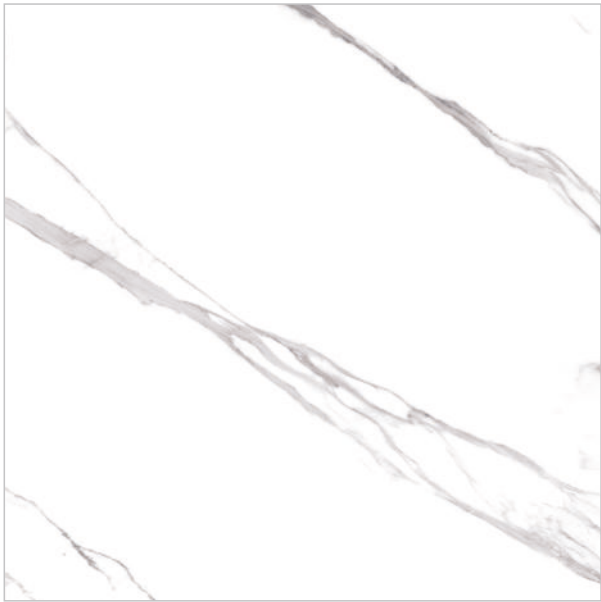
Statuario Classic
