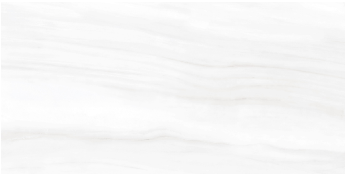
Eldorado Bianco
