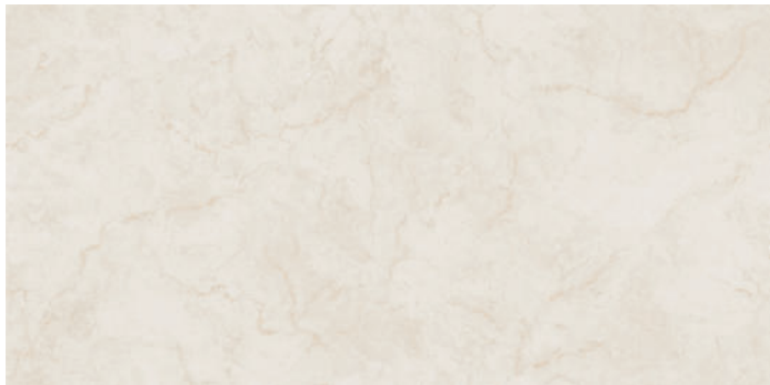
Marfil
