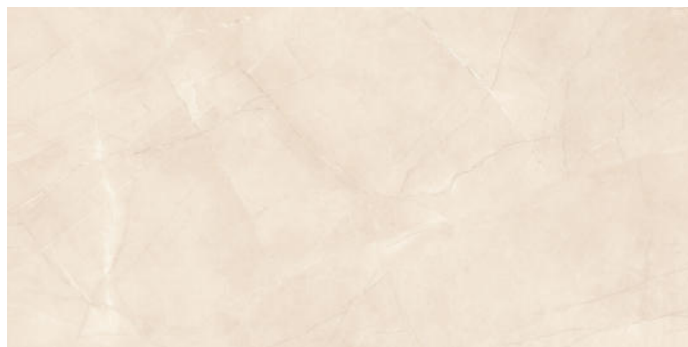
Oracle Beige
