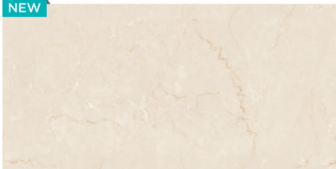
Andrix Beige
