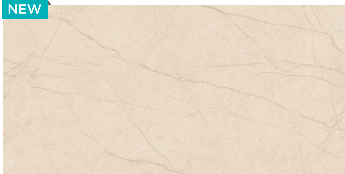
Levica Beige
