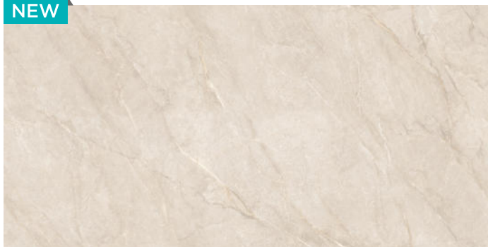
Genetta Beige
