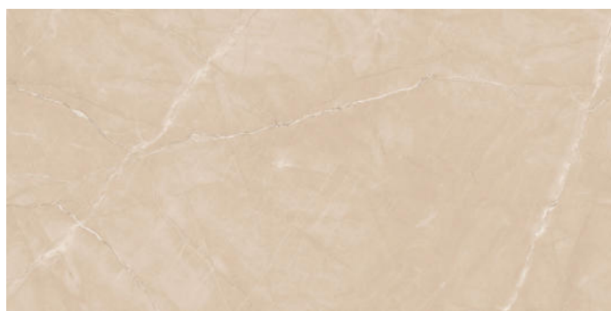
Liston Beige
