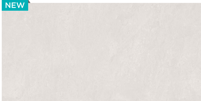
Panora Gris
