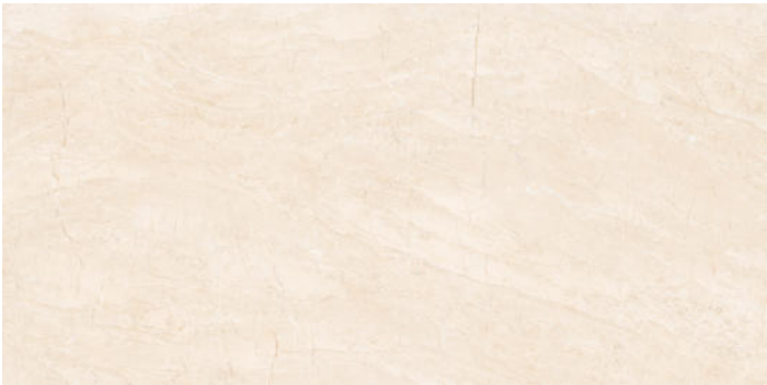
Fantasia Beige
