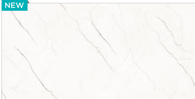
Pelica Statuario
